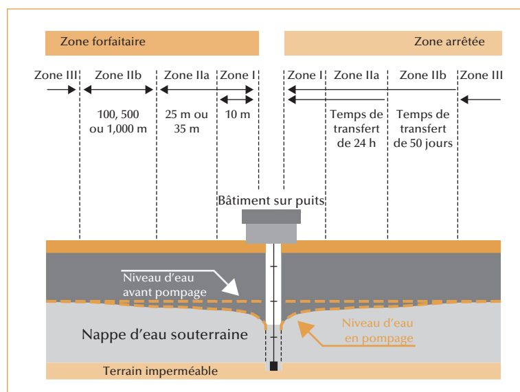
Figure 5 – Zones de protection des captages.
