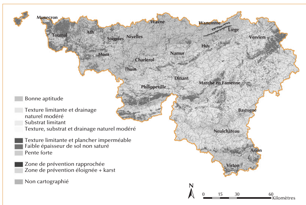
Figure 9 – Carte d'aptitude du sol à l'évacuation souterraine des eaux usées traitées pour la région wallonne.
