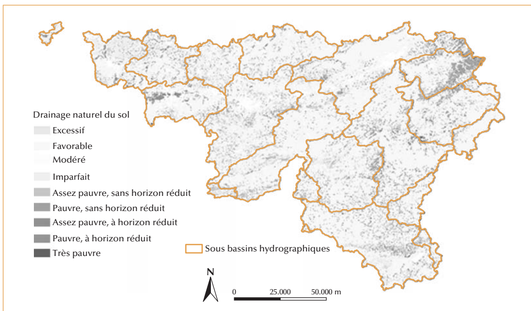
▲ Figure 4 – Classes de drainage naturel en région wallonne.
