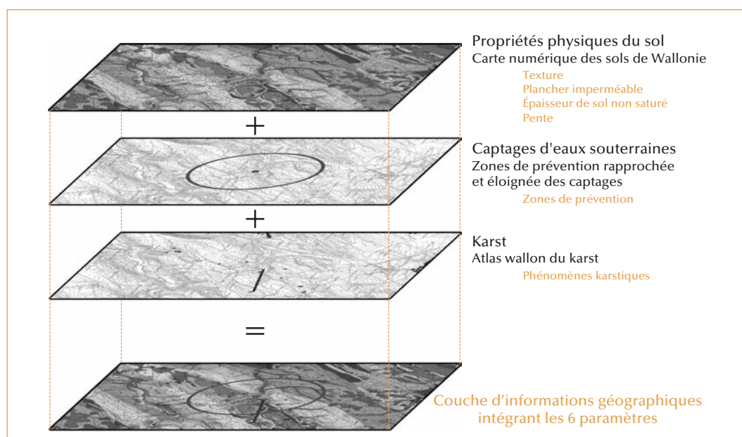
◀ Figure 1 – Prétraitement cartographique pour l'intégration des 6 paramètres retenus.
